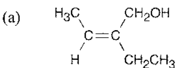
(Z)-2-Ethyl-2-buten-1-ol
