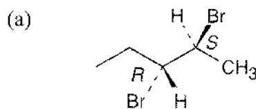
(2 S ,3 R )-2,3-Dibromopentane
