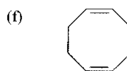
1,5-Cyclooctadiene
