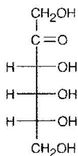
D-Psicose
