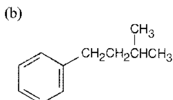
(3-Methylbutyl)benzene
