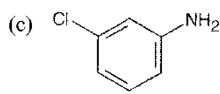
m -Chloroaniline
