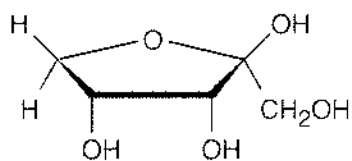
\beta -D-Ribulofuranose
