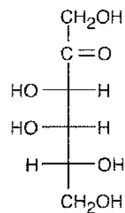
D-Tagatose
