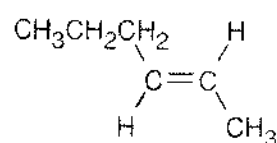
(E)-2-Hexene
