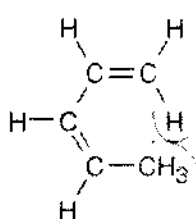
cis -1,3-Pentadiene
