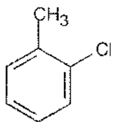
o -Chlorotoluene
