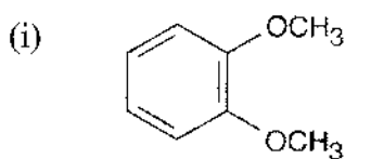
o -Dimethoxybenzene
