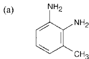
3-Methyl-1,2-benzenediamine
