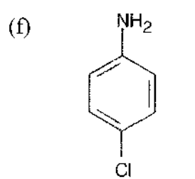
p -Chloroaniline
