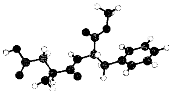
Aspartame
