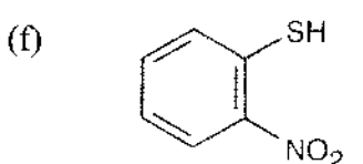
o -Nitrobenzenethiol
