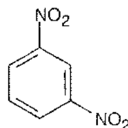
m -Dinitrobenzene
