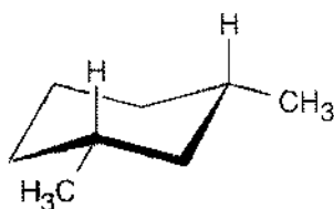
cis -1,3-Dimethylcyclohexane
