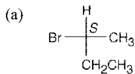
(S)-2-Bromobutane CH 3 CH 2 CH(Br)CH 3
