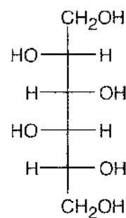
Iditol
