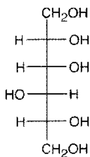
Gulitol
