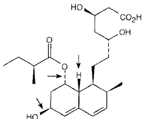
Pravastatin (Pravachol)
