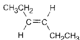
(E)-3-Hexene
