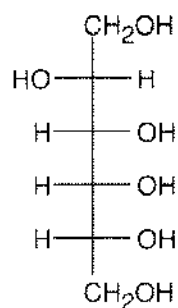
Altritol
