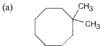
1,1-Dimethylcyclooctane
