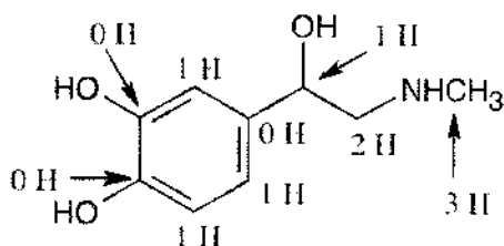
Adrenaline – C_9H_{13}NO_3
