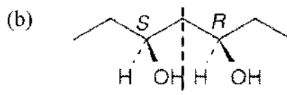
meso -3,5-Heptanediol
