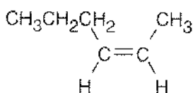
(Z)-2-Hexene
