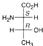
L-Threonine
