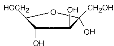
\alpha -D-Fructofuranose
