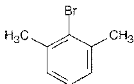
2-Bromo-1,3-dimethylbenzene
