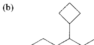
3-Cyclobutylhexane
