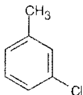
m -Chlorotoluene
