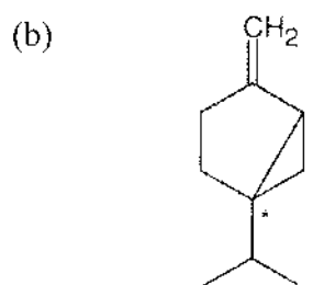
Sabinene
