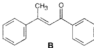
Dypnone (sunscreen)
