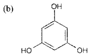
1,3,5-Benzenetriol
