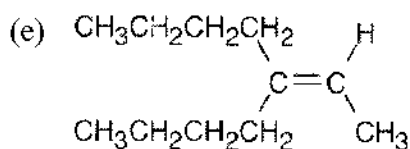
3-Butyl-2-heptene
