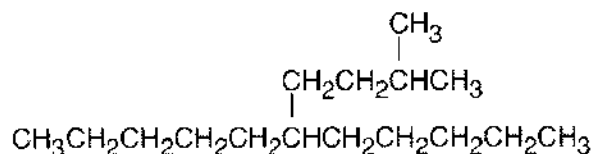
6-(3-Methylbutyl)-undecane
