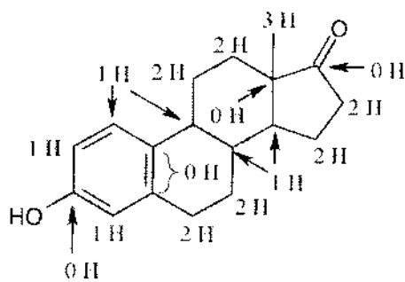
Estrone – C_{18}H_{22}O_2
