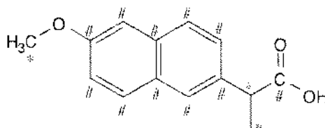
Naproxen
