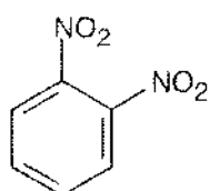
o -Dinitrobenzene
