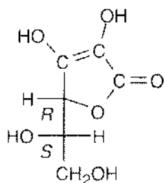
L-Ascorbic acid
