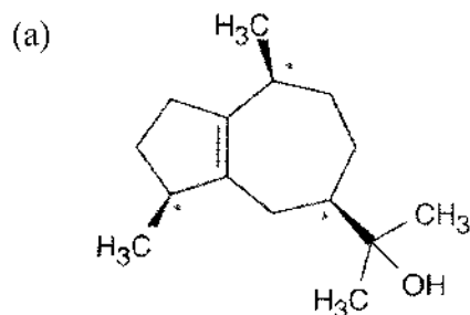
Guaiol
