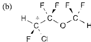
Enflurane
