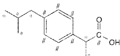
Ibuprofen
