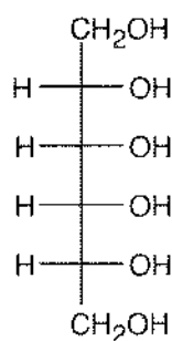
Allitol
