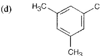
1-Chloro-3,5-dimethylbenzene
