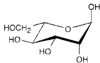
\alpha -L-Mannopyranose
