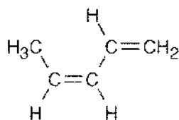
cis -1,3-Pentadiene
