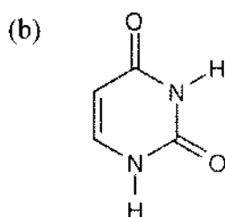
Uracil (U) RNA
